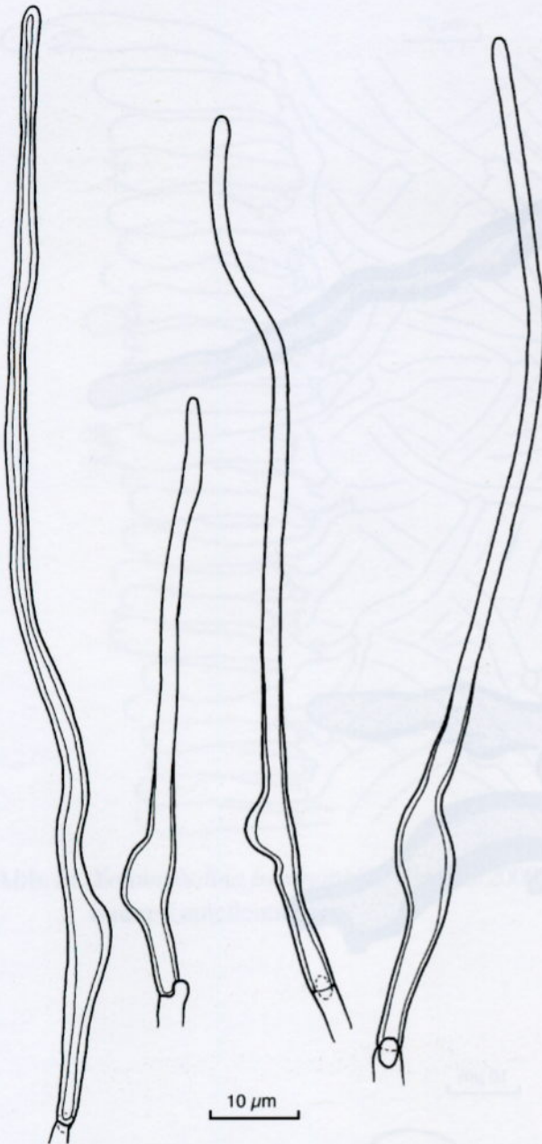
Abb. 6: Xeromphalina fraxinophila , CH 273/2000, Cystiden der Rhizomorphenoberfläche
