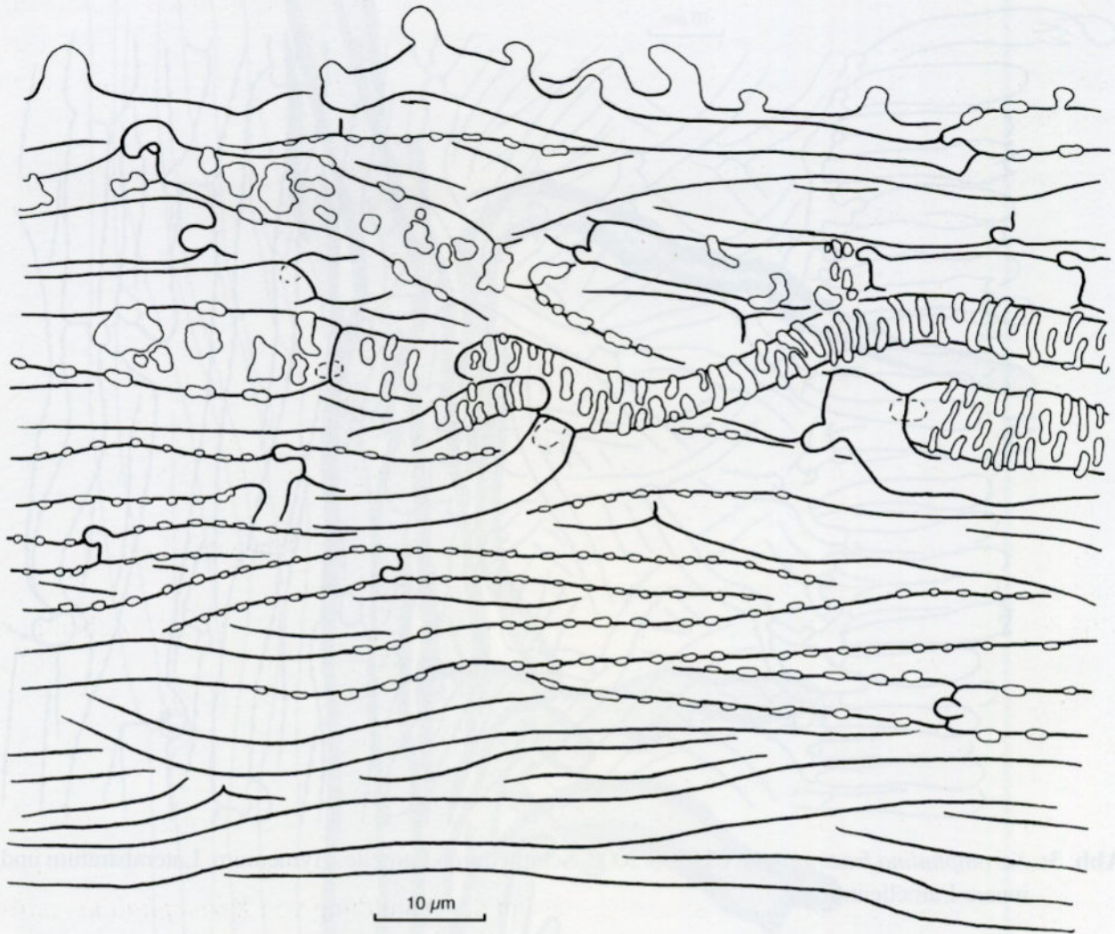
Abb 1: Xeromphalina fraxinophila , CH 273/2000, Hutdeckschicht
