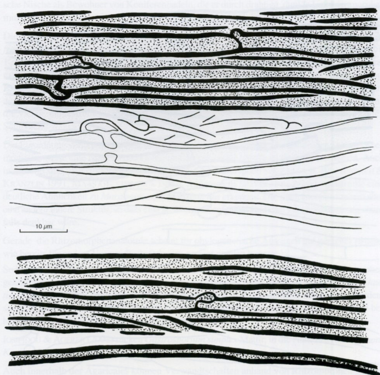
Abb. 7: Xeromphalina fraxinophila , CH 273/2000, Rhizomorphe im Schnitt; unten mit von der Rhizomorphe abgesetztem Hals einer Cystide
