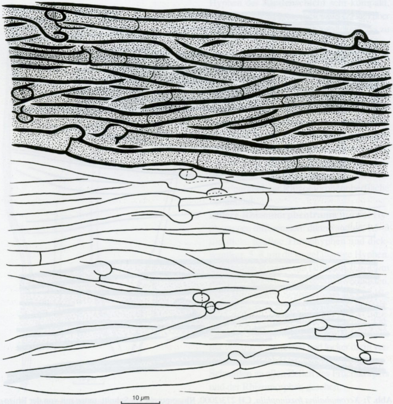
Abb. 8: Marasmiellus perforans , CH 491/2000, Rhizomorpe im Schnitt
