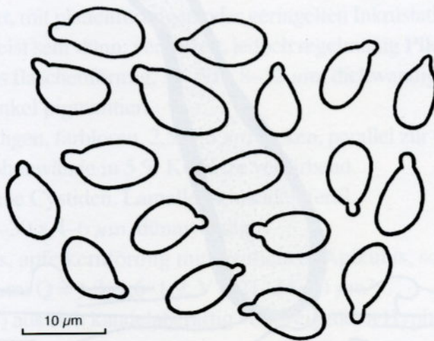
Abb. 4: Xeromphalina fraxinophila , CH 273/2000, Sporen
